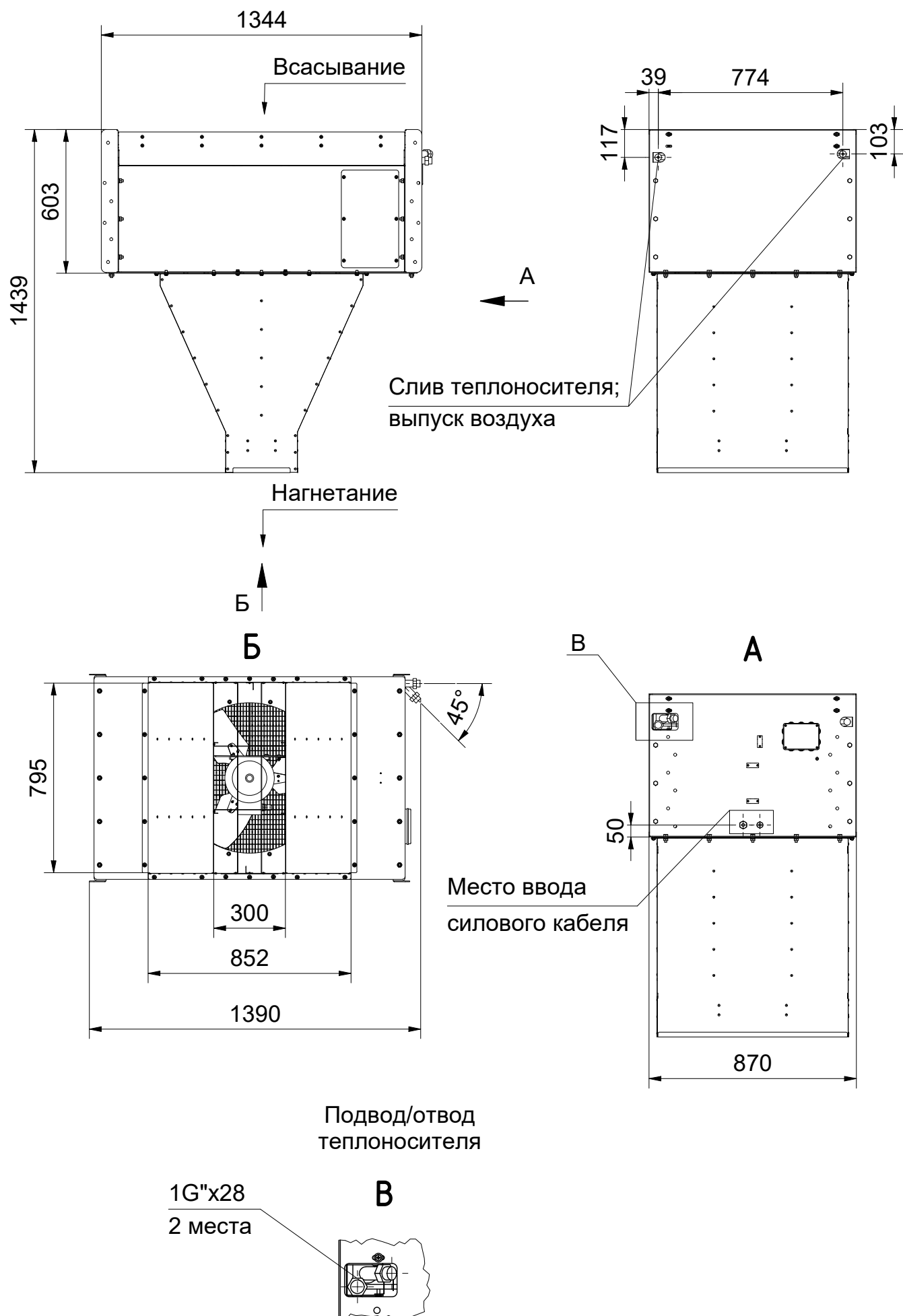
Рисунок 4. Габаритные и присоединительные размеры
