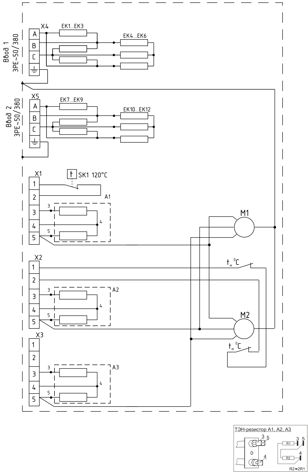
Рисунок 4. Электрическая схема завесы КЭВ-42П7011Е
