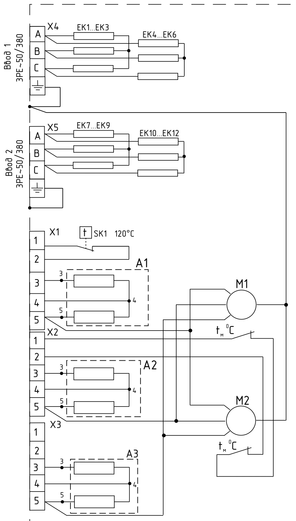
Рисунок 3. Электрическая схема занесы КЭВ-24П7011Е, КЭВ-36П7011Е
