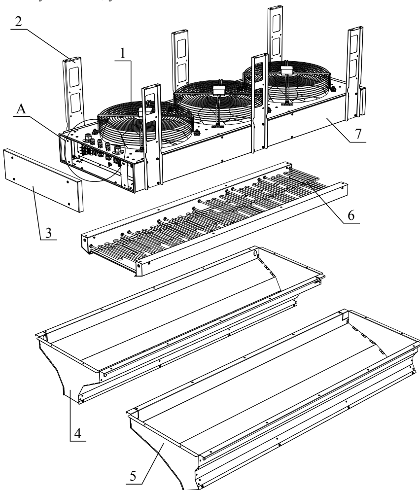
Рисунок 1. Воздушно-тепловая завеса
