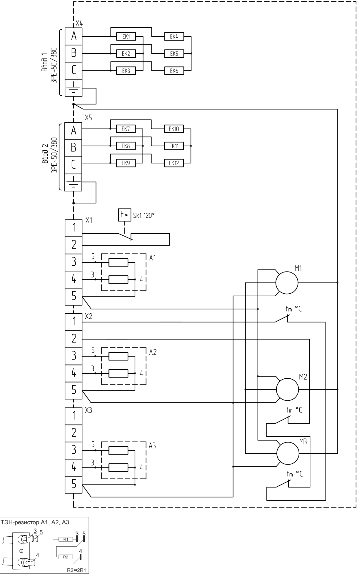
Рисунок 5. Электрическая схема завесы КЭВ-36П7021Е
