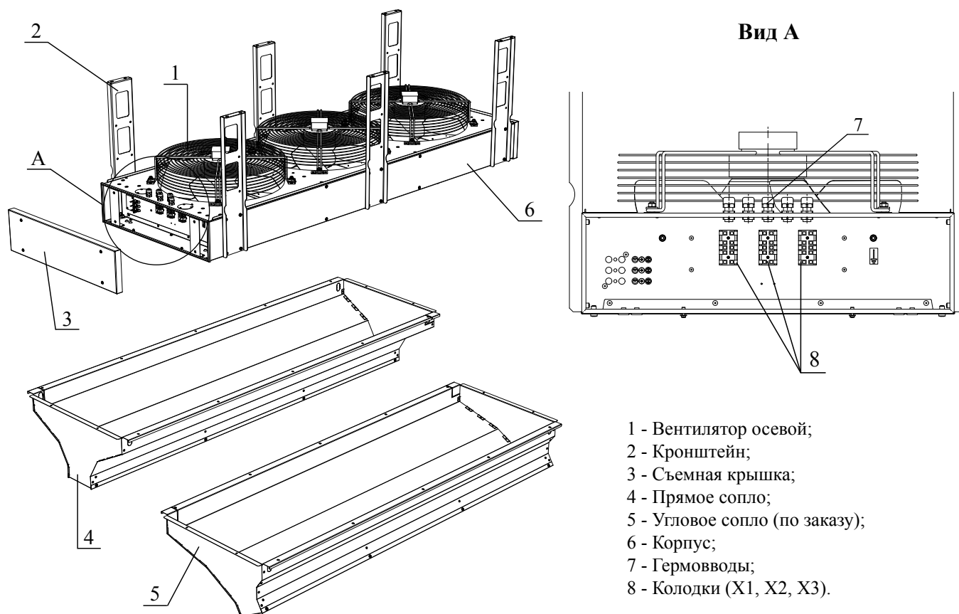
Рисунок 1. Воздушная завеса
