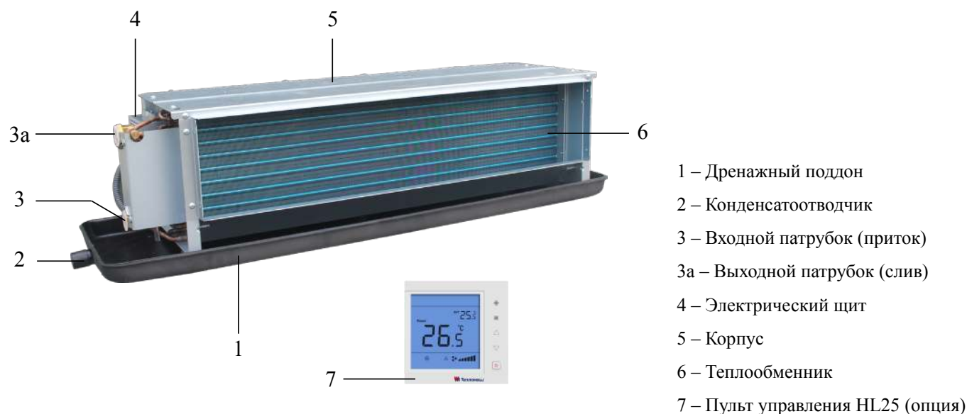
Рисунок 1. Фанкойл кассетный
